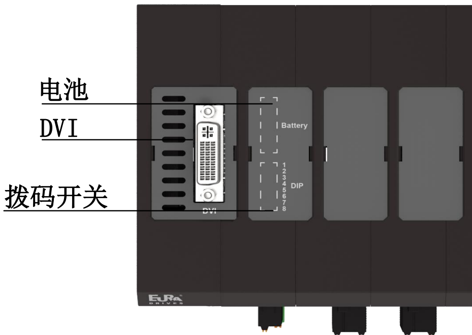
运动控制器整体视图及结构名称
